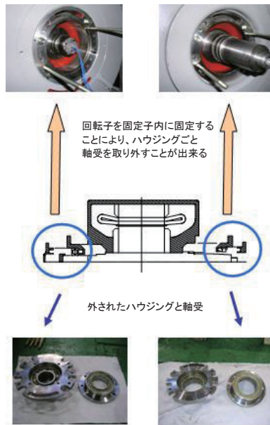
軸受交換構造
