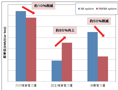
消費電力量測定結果
